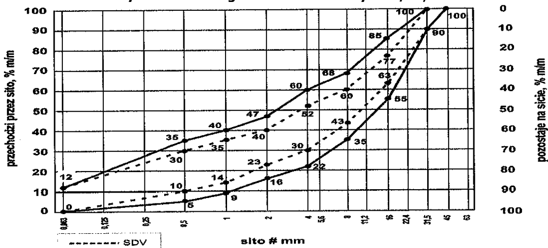
Rys1. Pole dobrego uziarnienia kruszywa 0/31,5
