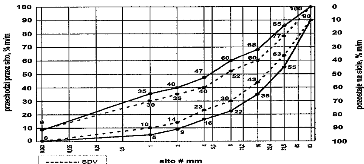
Rys.2 Mieszanka kruszywa 0/63
