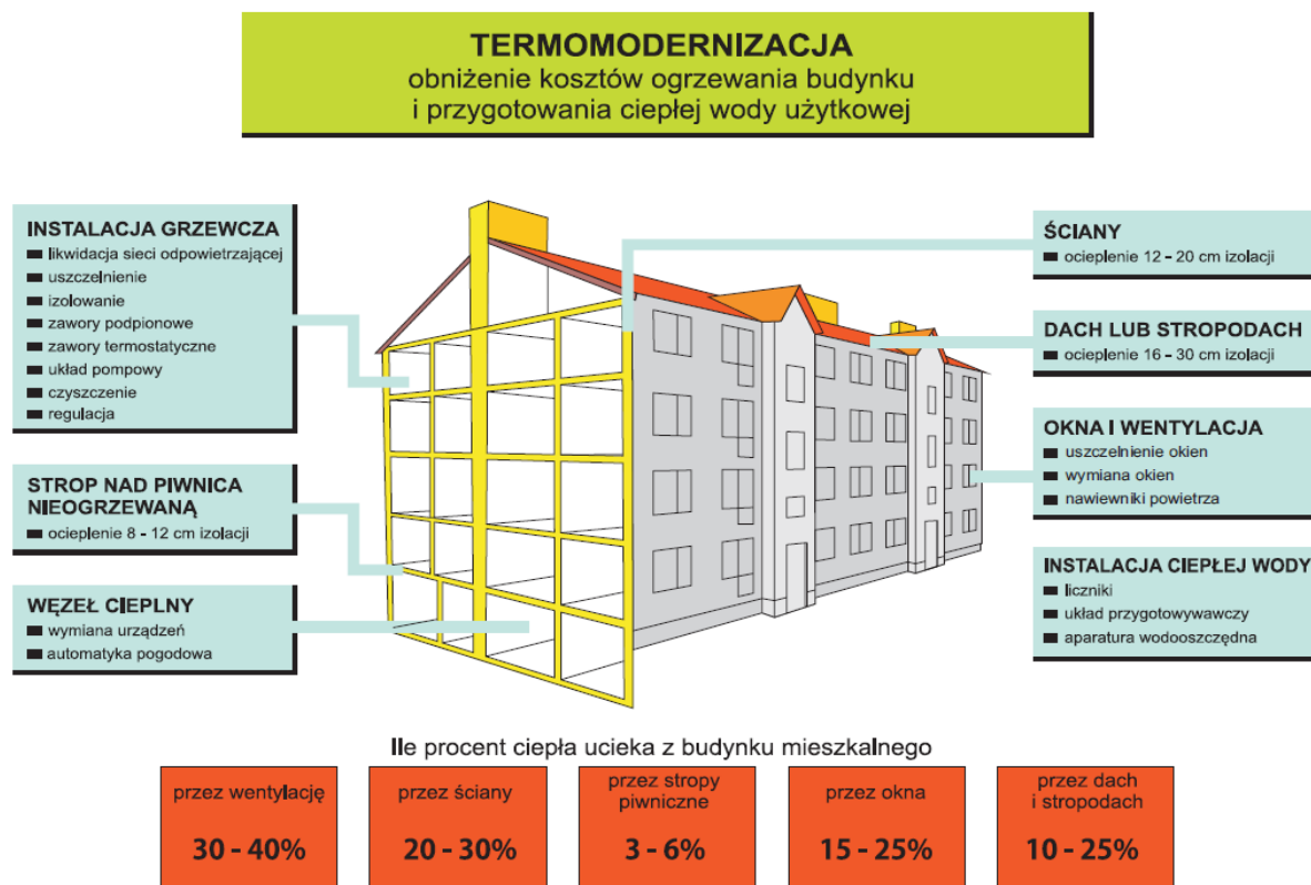
Ryc. 9. Termomodernizacja budynku
