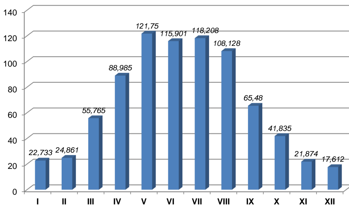
Wykres 3. Natężenie promieniowania słonecznego (kWh/m 2 ) dla poszczególnych miesięcy dla typowego roku meteorologicznego dla stacji meteorologicznej w Chojnicach
