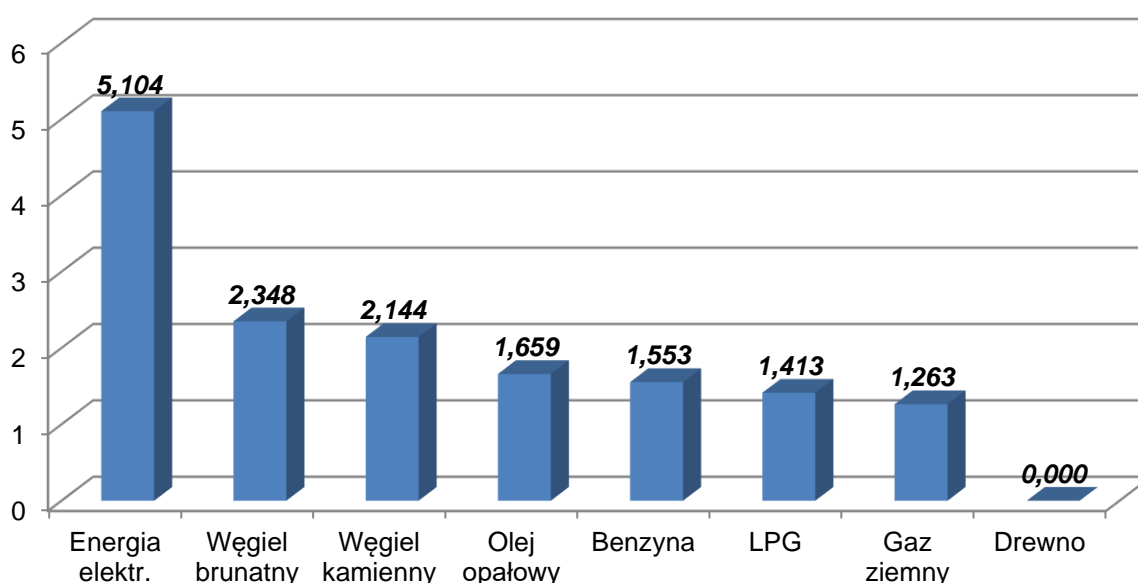
Wykres 23. Emisja CO 2 z poszczególnych nośników energii (w przeliczeniu na ekwiwalent wartości opałowej 1 Mg węgla kamiennego) (MgCO 2 /22,63 GJ)
