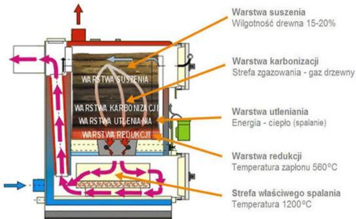
Ryc. 20. Schemat spalania drewna w kotle zgazowującym
