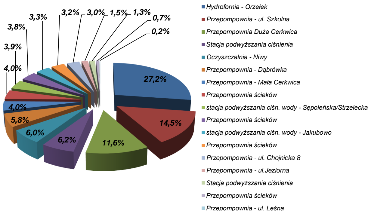
Wykres 21. Udział w zużyciu energii elektrycznej poszczególnych obiektów infrastruktury wodno-kanalizacyjnej
